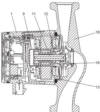
1-сур. ALPHA2 L сорғысының кесірі
