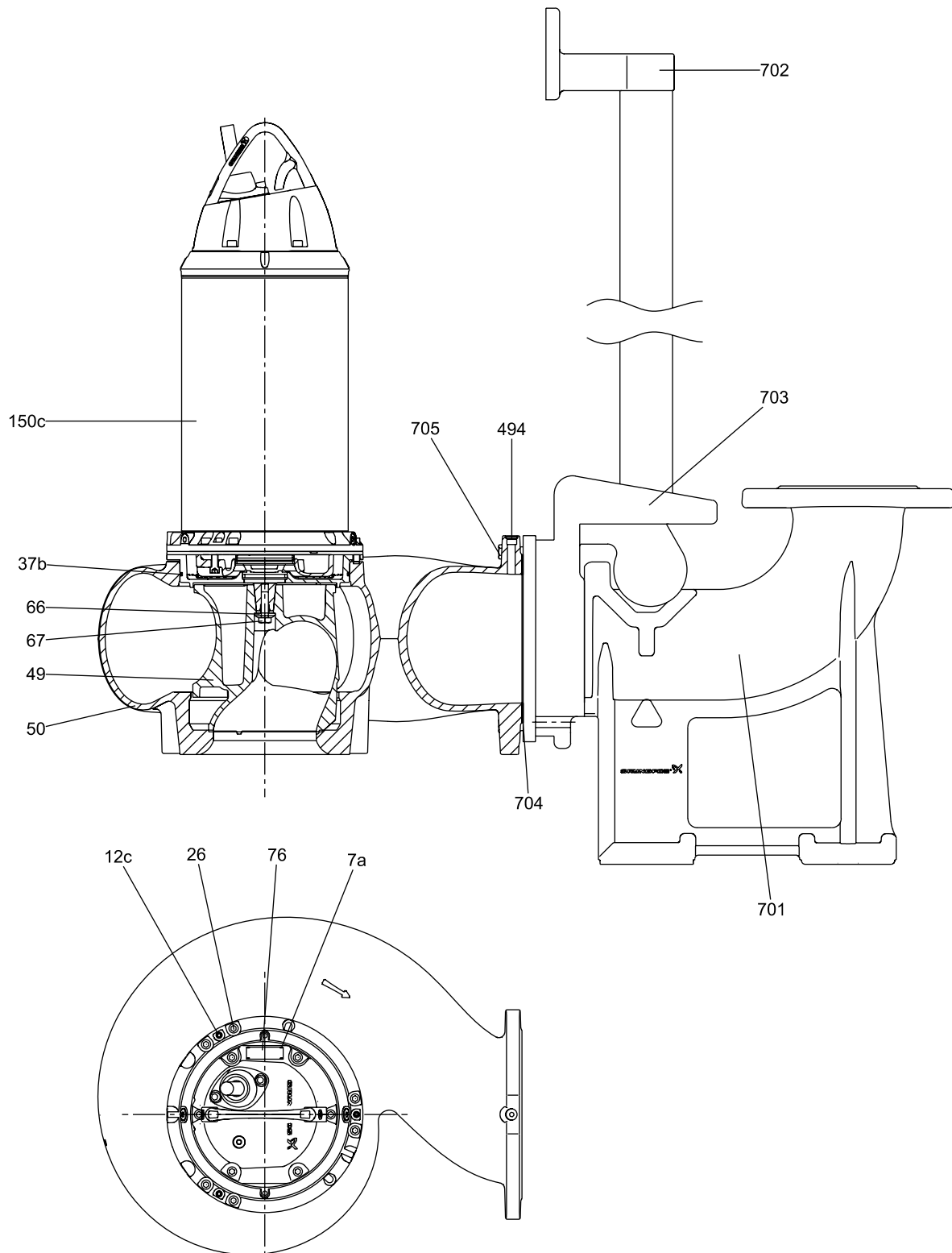
Рис. 12 Насос SE/SL с направляющими клыками для автоматической трубной полумуфты
