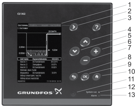
Рис. 17 Панель управления CU 362
