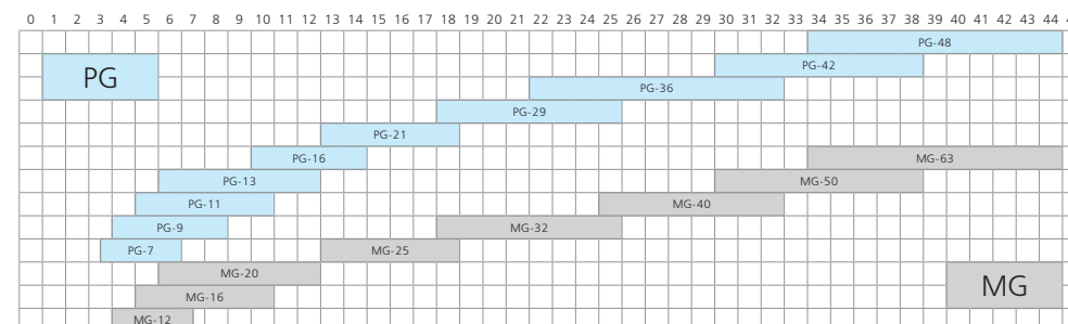
Размеры кабелей, фиксируемые в кабельных вводах с резьбой PG и метрической резьбой
